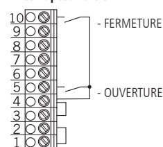
Interrupteur à clé
