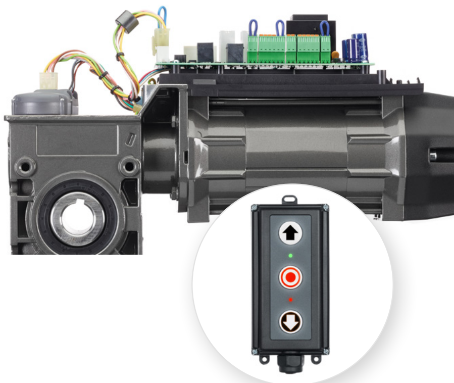
Commutateur CS-I-15
