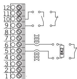
Entrée 1 (9 + 10) Barre palpeuse 8,2 kΩ / DW (5+6)
