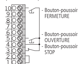
Bouton-poussoir OUVERTURE / STOP / FERMETURE (solution à 4 fils)
